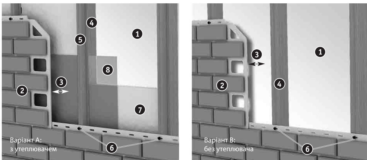
1 – стіна будинку, 2 – фасадна панель, 3 – вентиляований зазор, 4 – рейка 50x50 мм, 5 – рейка 25x25 мм, 6 – шуруп, 7 – утеплювач, 8 – гідроізолююча плівка
